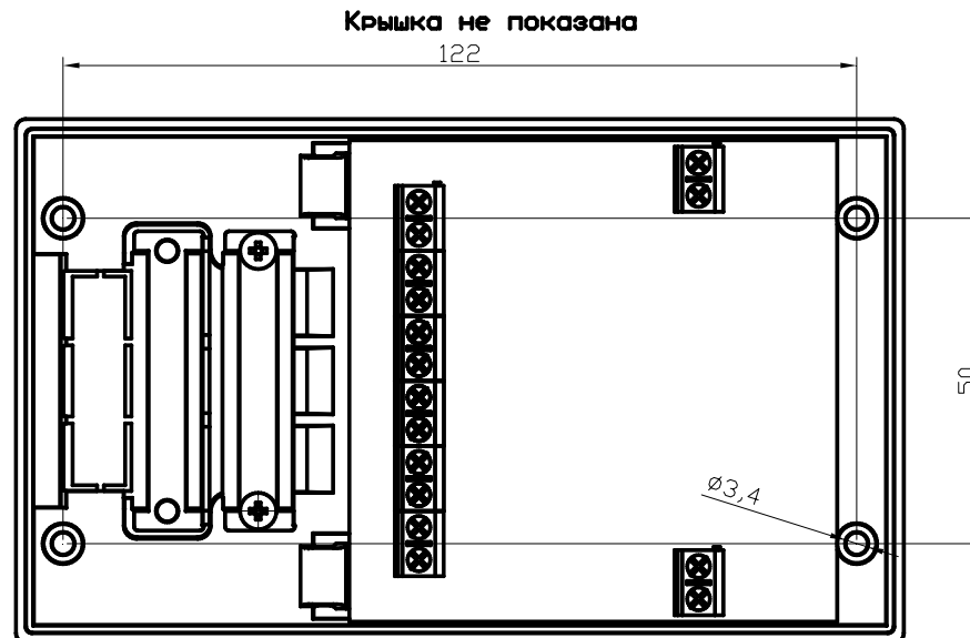
Рис.2 Установочные размеры блока сопряжения ADC248-1
