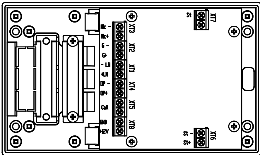
Рис.1 Внешний вид блока сопряжения ADC248-1
