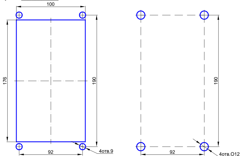
Рис1. Разметка под крепление DP7000ip-Hybrid/PCVBS а) снаружи; б) изнутри.
