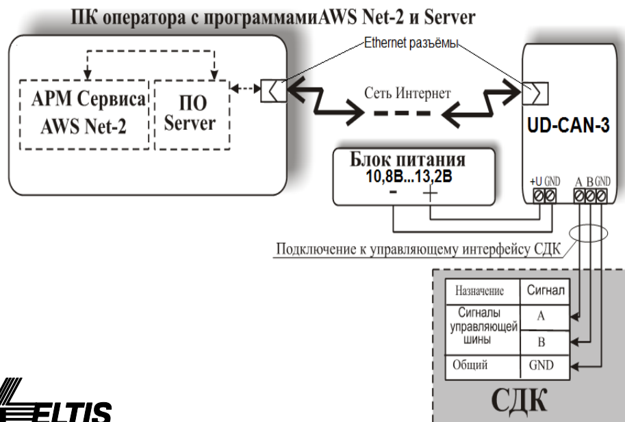
Рис.3 Схема подключения устройства сопряжения UD-CAN-3 Производитель: ЭЛТИС, Россия
