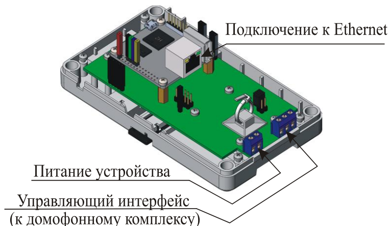
Рис.1 Вид устройства сопряжения со снятой крышкой
