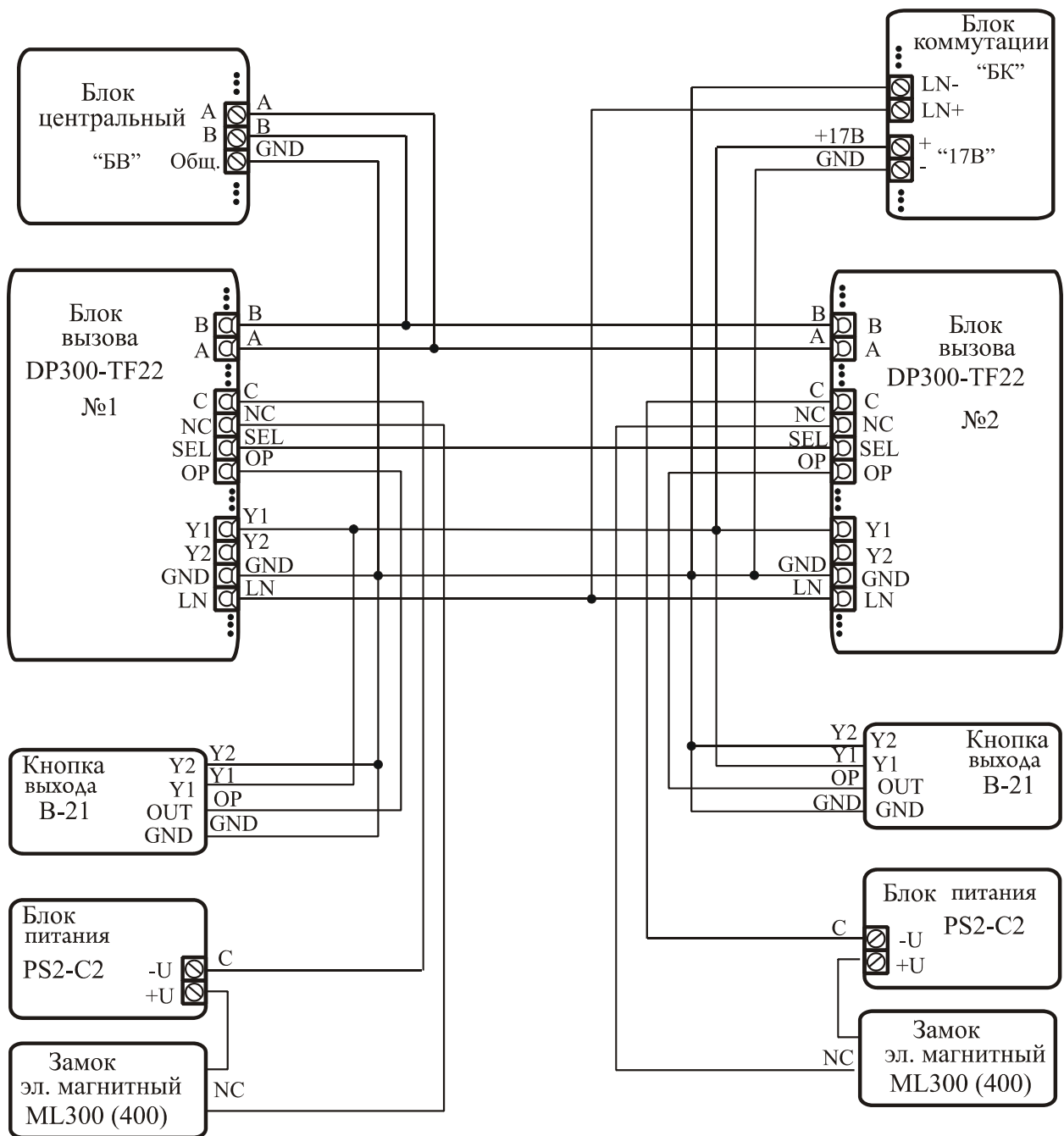
Рис.3 Пример схемы подключения DP300-TF22 в составе прибора «Форпост».
