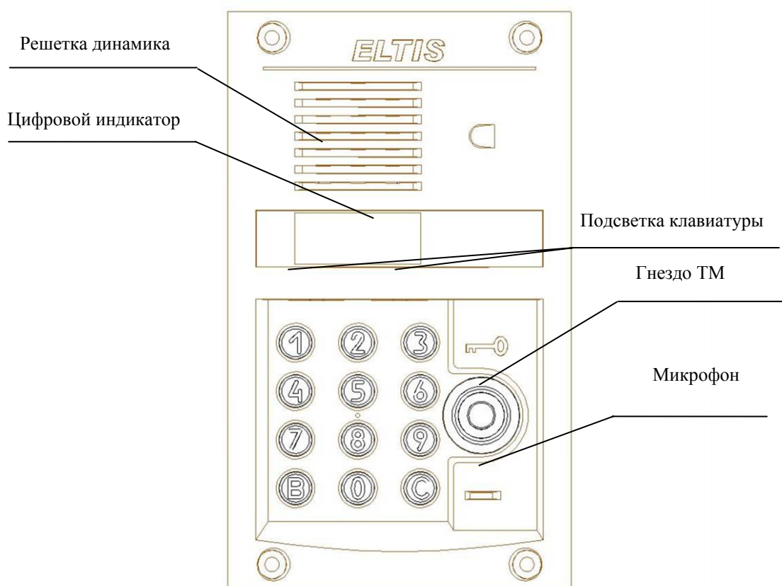
Рис.1 Внешний вид со стороны лицевой панели блока вызова DP300-TF22.
