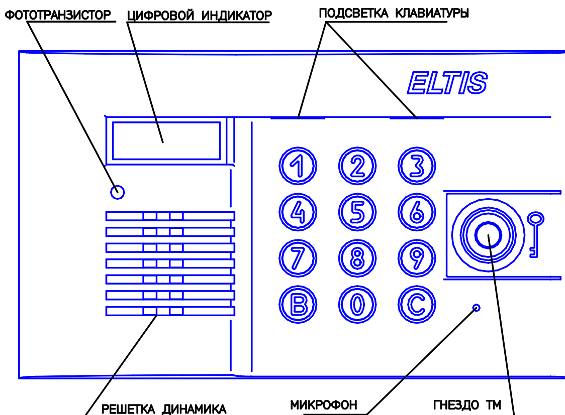
Рис.1 Внешний вид со стороны лицевой панели блока вызова DP400-TD12
