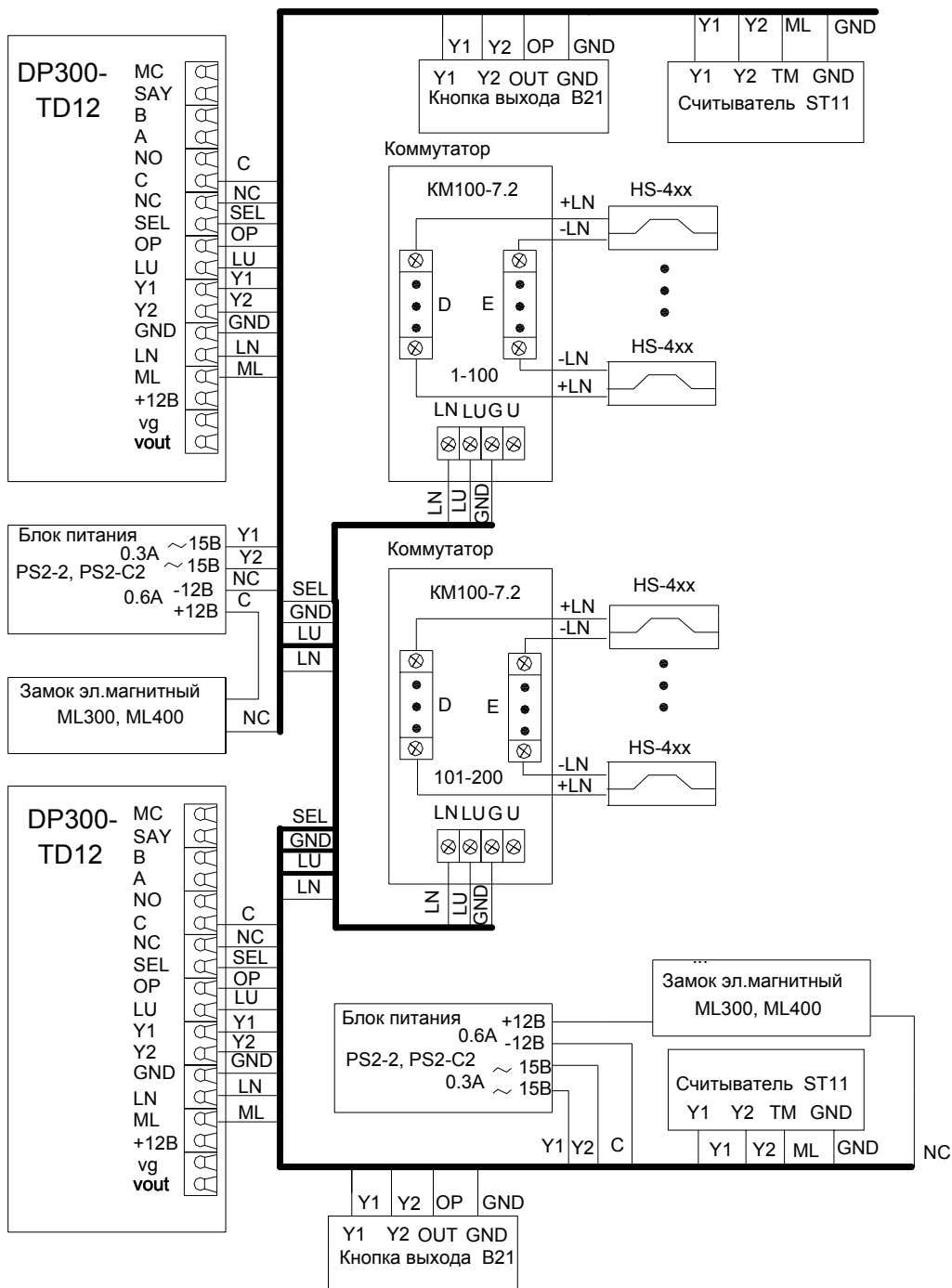
Рис.3 Пример схемы подключения DP300-TD12 в составе домофонного комплекса.
