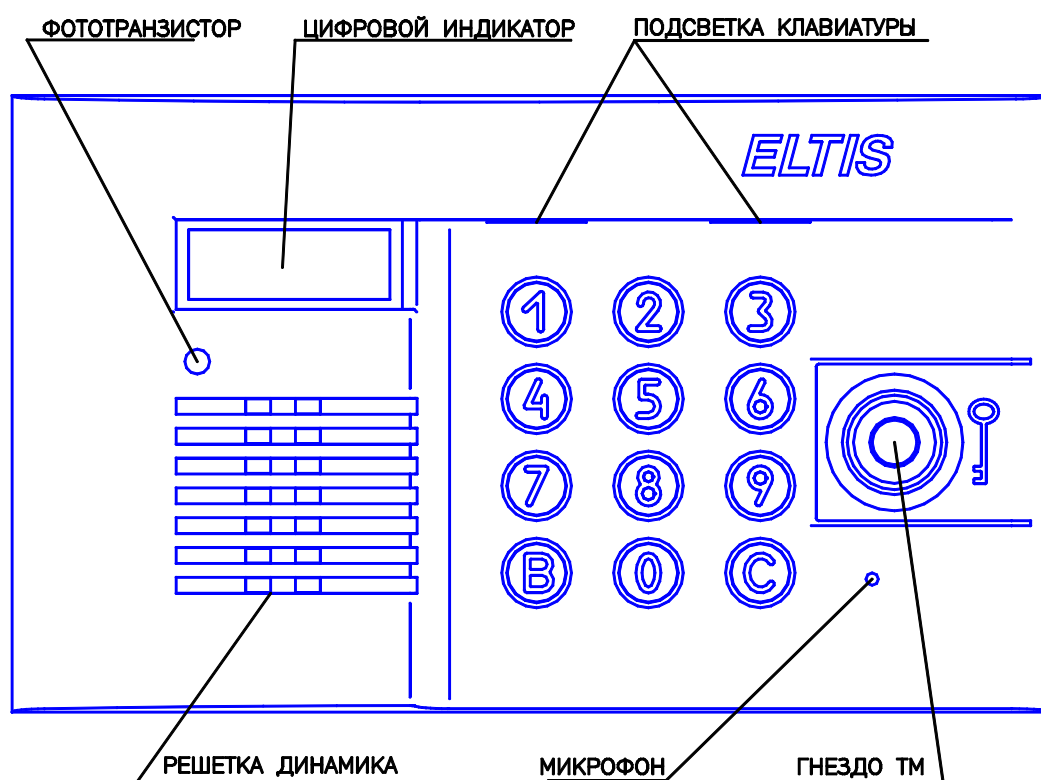
Рис.1 Внешний вид со стороны лицевой панели блока вызова DP300-TD12.
