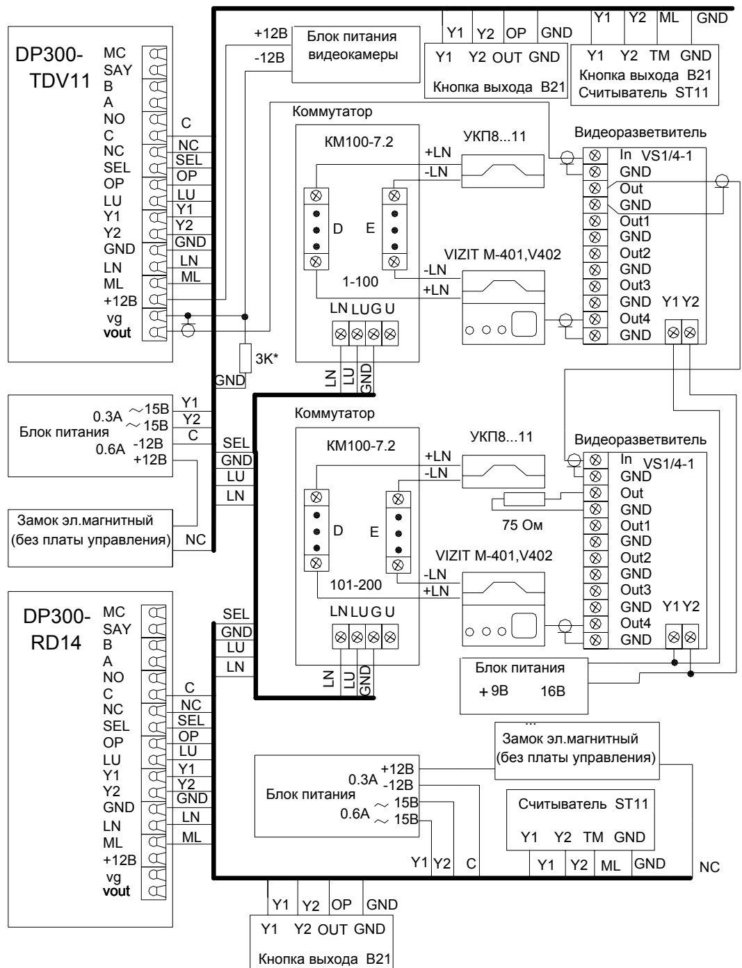
Рис.3 Пример схемы подключения DP300-RD14 и DP300-TDV11 в составе домофонного комплекса.
