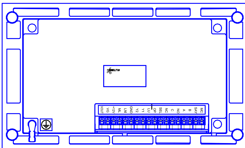
Рис.1 Внешний вид со стороны лицевой панели блока вызова DP300-RD14.
