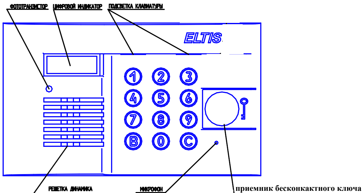
Рис.1 Внешний вид со стороны лицевой панели блока вызова DP300-RD14.
