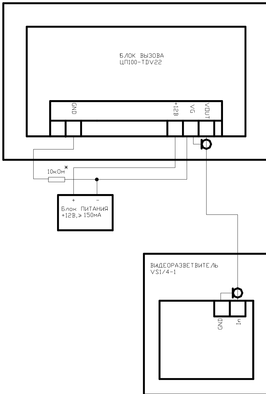
Рис.4 Схема подключения блока вызова с видеокамерой.
