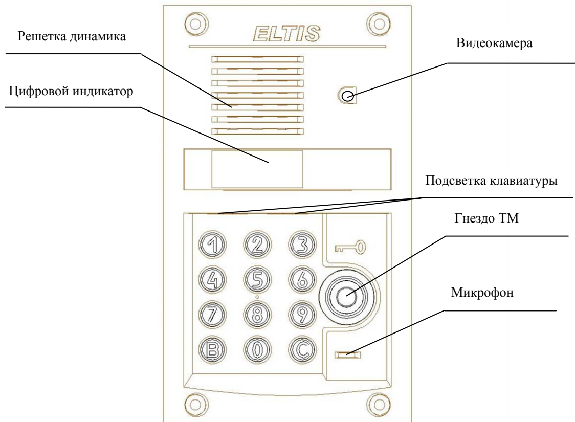
Рис.1 Внешний вид со стороны лицевой панели блока вызова ЦП100-TDV22.
