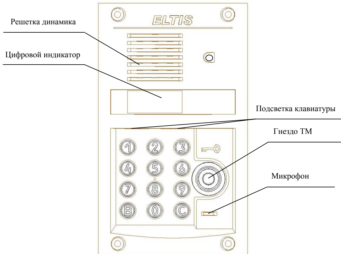
Рис.1 Внешний вид со стороны лицевой панели блока вызова ЦП100-TD22.
