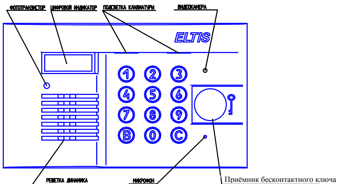
Рис.1 Внешний вид со стороны лицевой панели блока вызова ЦП100-RDV12.
