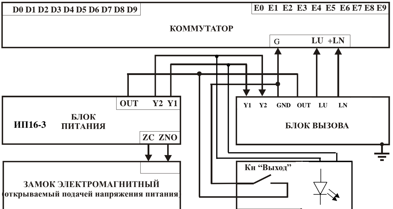
Рис.3 Схемы подключения различных типов замков, не имеющих собственной схемы управления.
