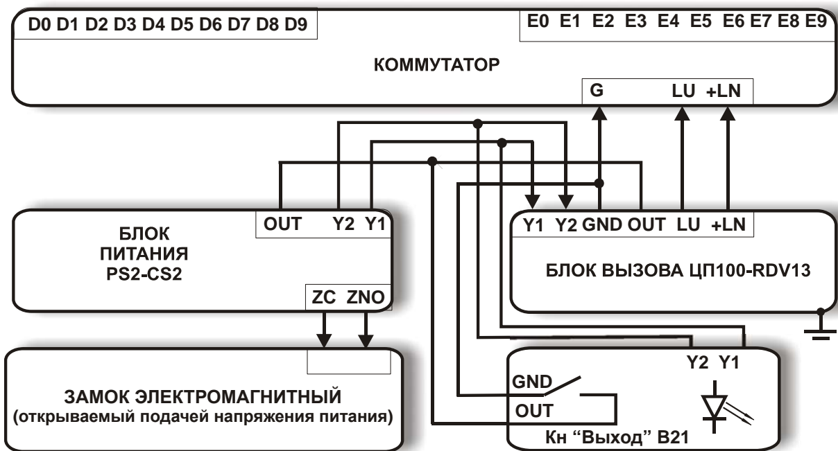
Рис.3 Схемы подключения различных типов замков, не имеющих собственной схемы управления.
