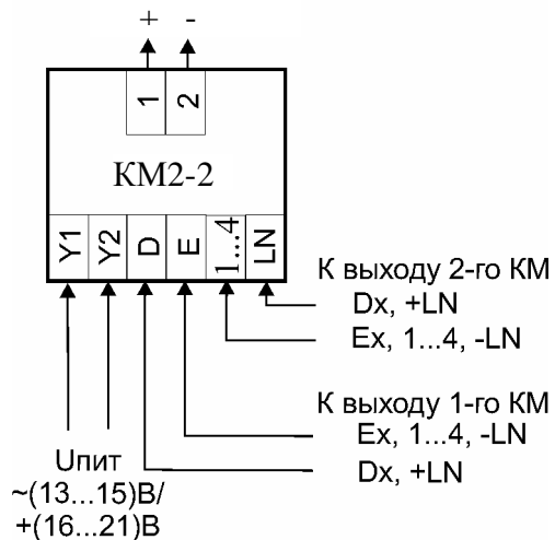
Рис. 5. Подключение дополнительного домофона через коммутатор КМ2
