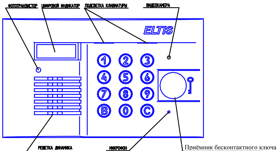
Рис.1 Внешний вид со стороны лицевой панели блока вызова ЦП100-RDV13.
