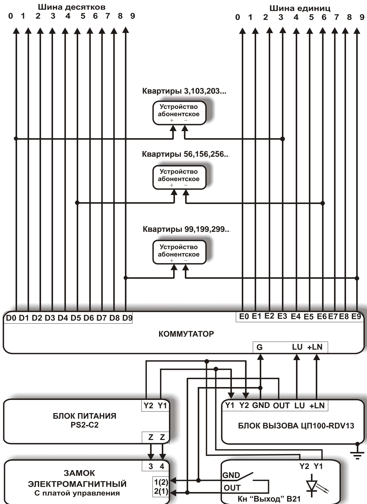
Рис. 2 Монтажная схема соединения блоков домофона.
