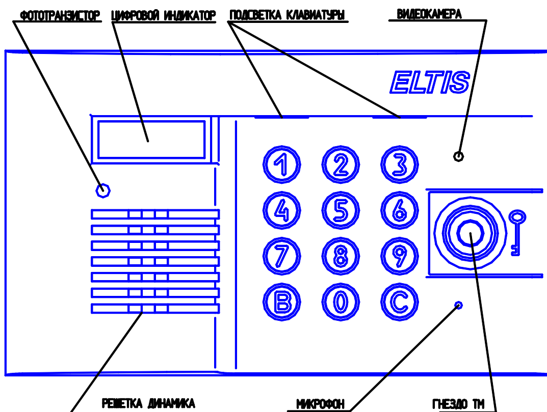
Рис.1 Внешний вид со стороны лицевой панели блока вызова DP400-TDV12
