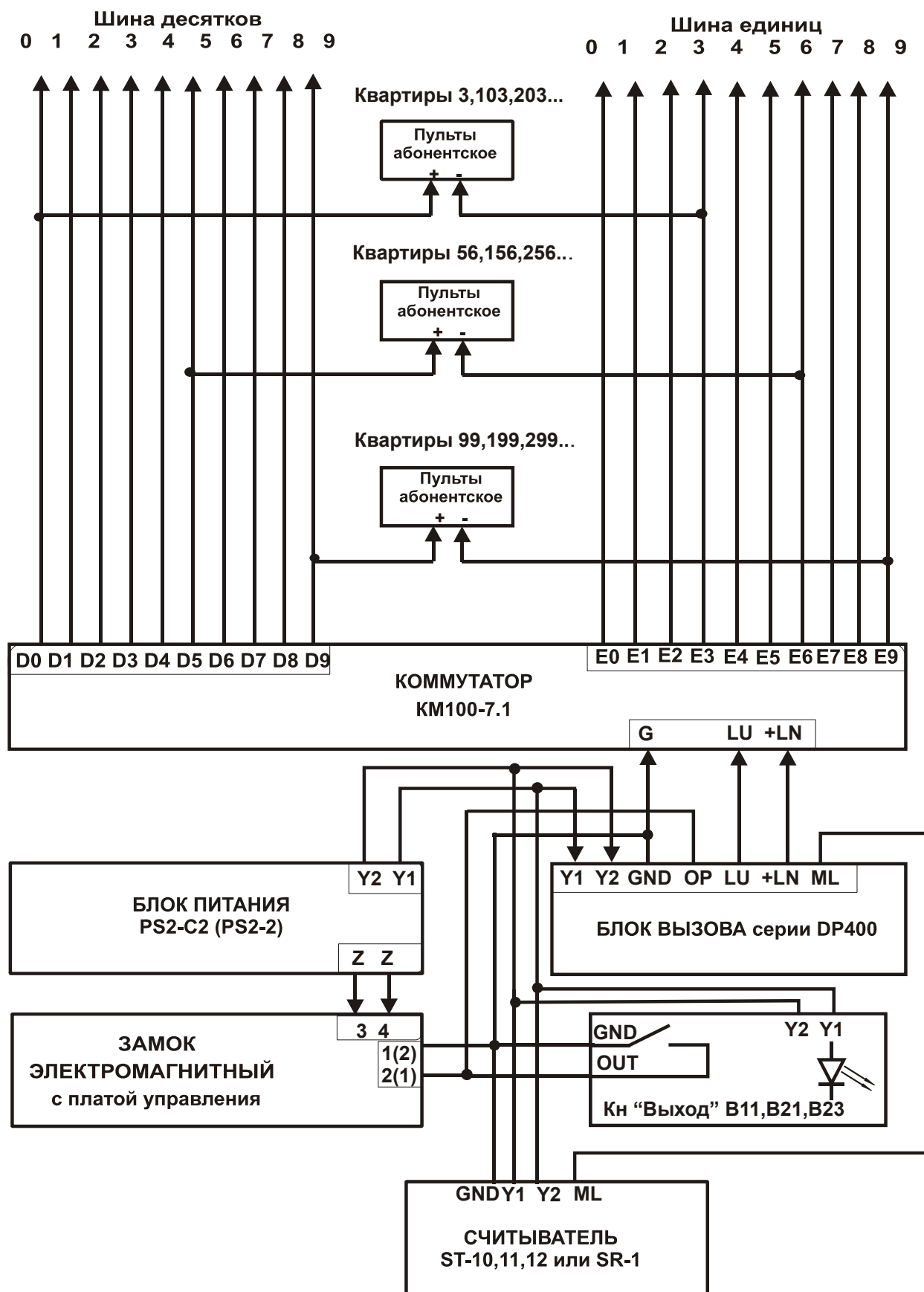
Рис. 3 Монтажная схема соединения блоков домофона (пример).
