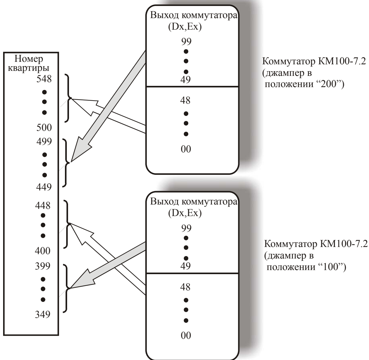
Рис.4 Пример схемы подключения двухсот квартир к двум коммутаторам КМ100-7.2. (Квартиры с 349 по 448)
