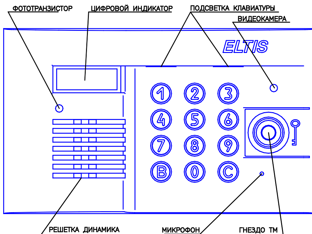
Рис.1 Внешний вид со стороны лицевой панели блока вызова DP300-TDV12.
