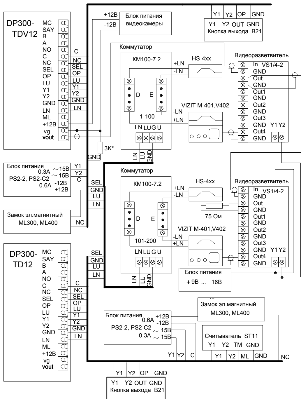
Рис.3 Пример схемы подключения DP300-TDV12 в составе домофонного комплекса.
