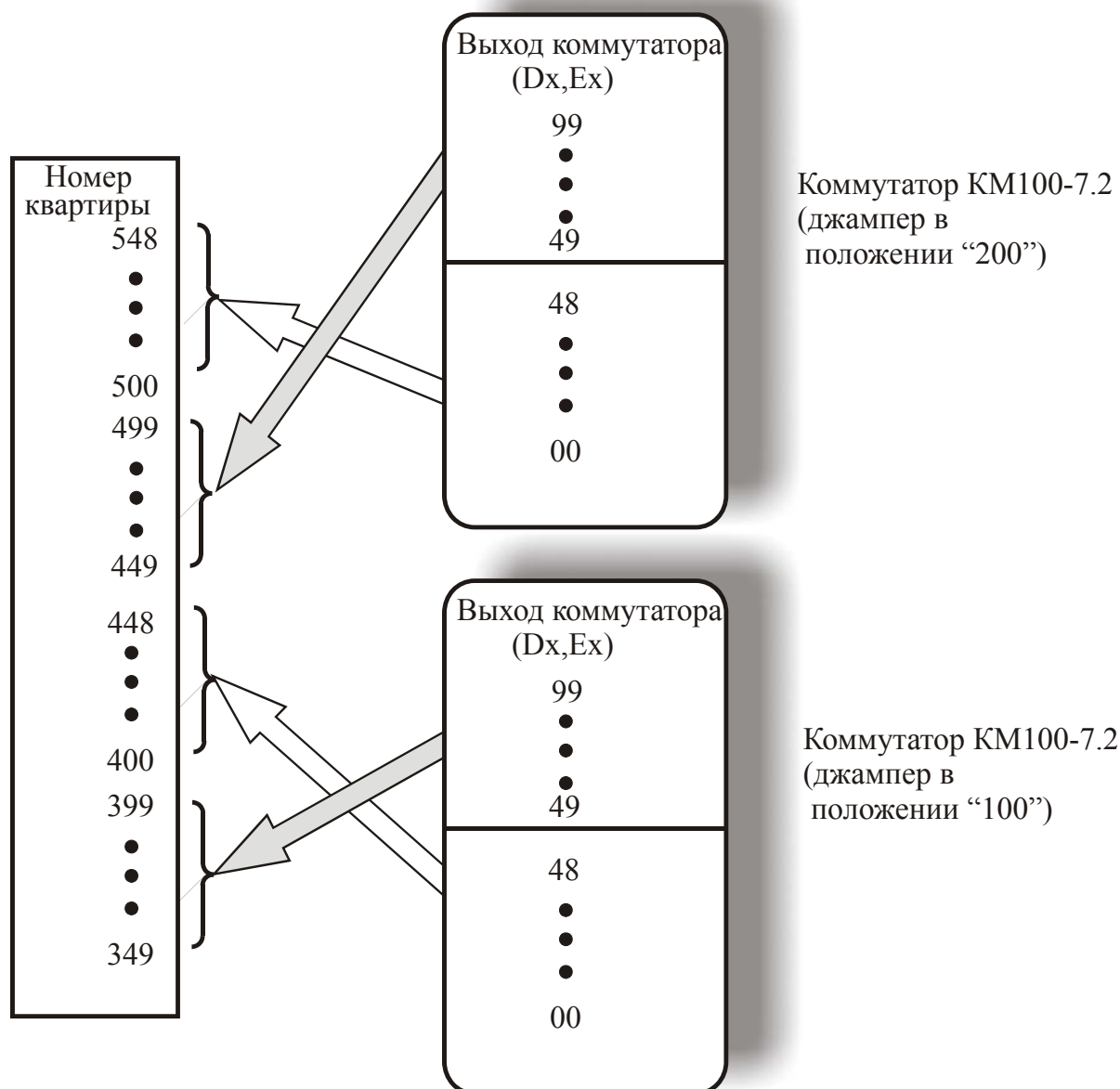
Рис.4 Пример схемы подключения двухсот квартир к двум коммутаторам КМ100-7.2. (Квартиры с 349 по 448)
