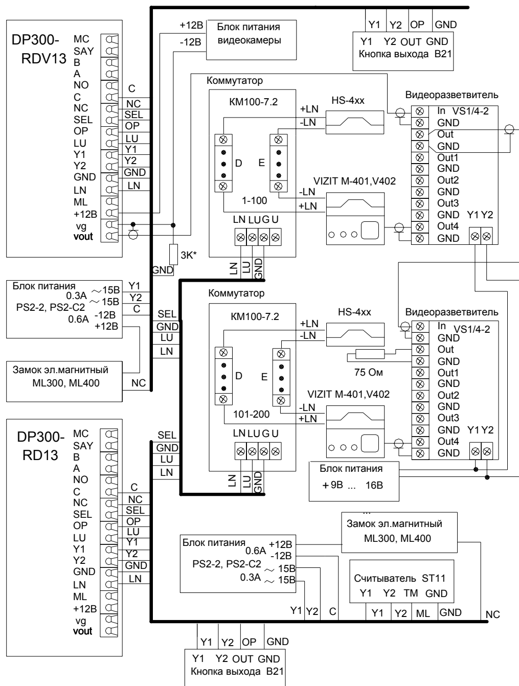
Рис.3 Пример схемы подключения DP300-RDV13 в составе домофонного комплекса.
