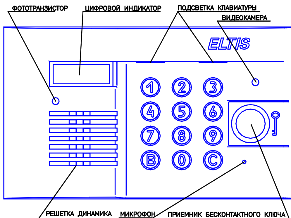
Рис.1 Внешний вид со стороны лицевой панели блока вызова DP300-RDV13.
